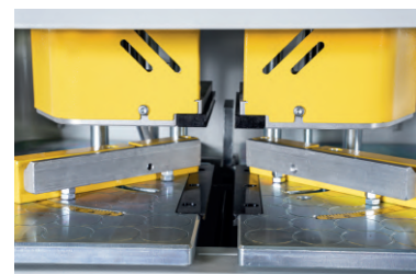
Cuchillas y topes ajustables
