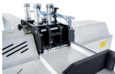
Corte de 2 perfiles a la vez
