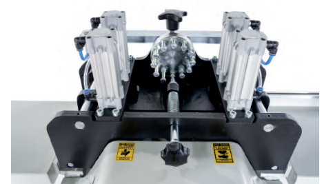
Sistema de rueda para 12 lamas diferentes
