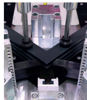
Pistones neumáticos
